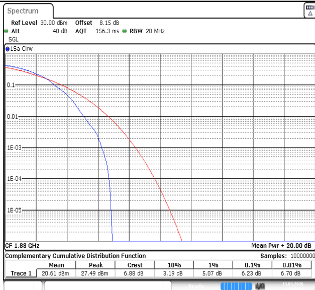
Band2-20MHz-QPSK-18900-1RB#0-PASS
