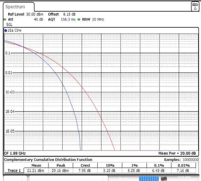
Band2-20MHz-QPSK-18900-100RB#0-PASS
