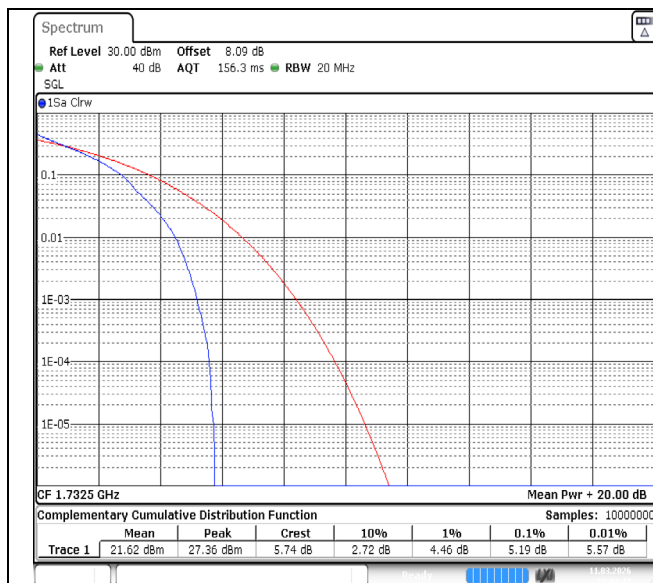
Band4-20MHz-QPSK-20175-1RB#0-PASS
