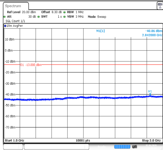
Band26(824-849)-1.4MHz-QPSK-26797-6RB#0-1000~3000-PASS
