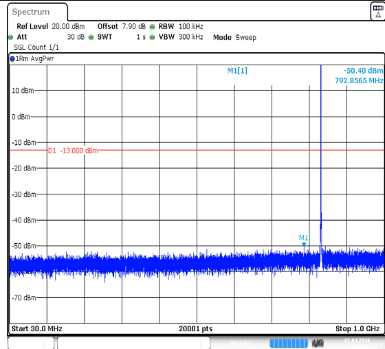
Band26(824-849)-1.4MHz-QPSK-26797-6RB#0-1000~3000-PASS
