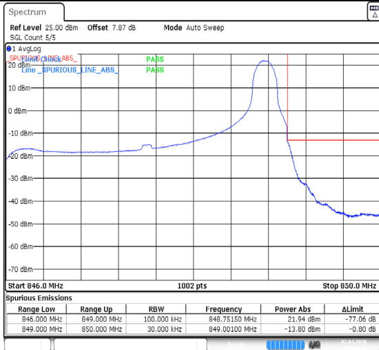
Band26(824-849)-3MHz-QPSK-26805-15RB#0-PASS
