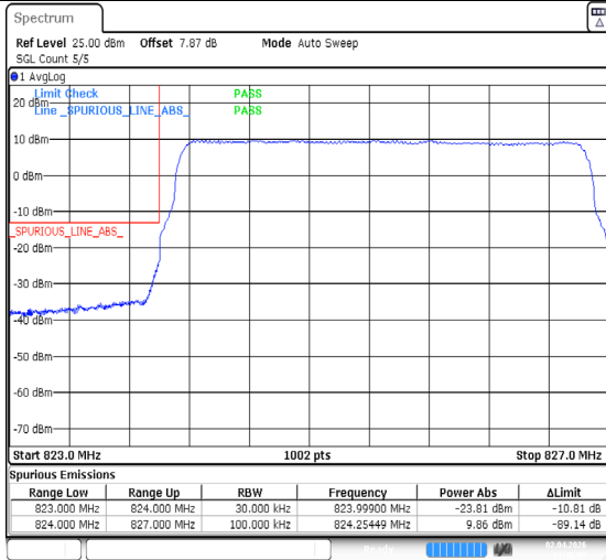
Band26(824-849)-3MHz-QPSK-26805-1RB#0-PASS
