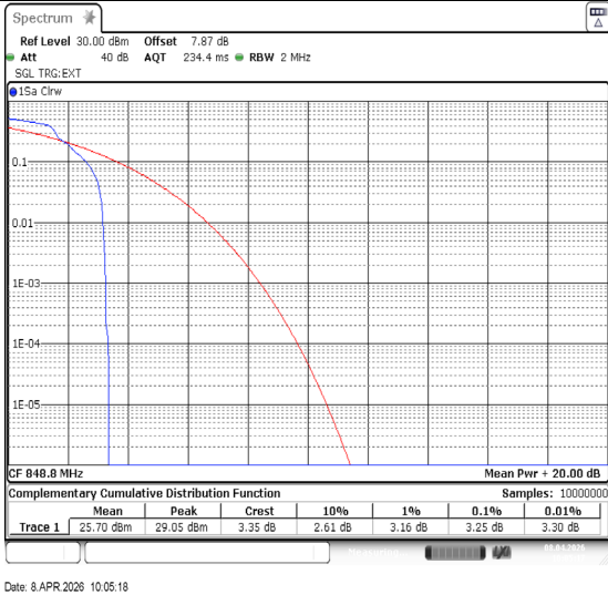
EGPRS850-251-8-PASS
