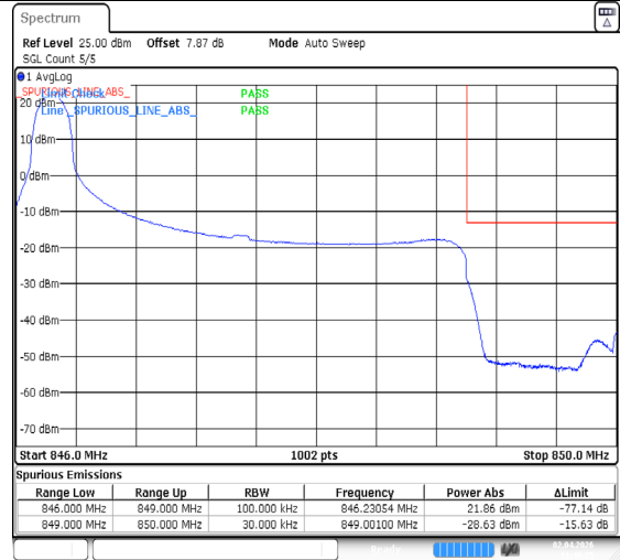
Band26(824-849)-3MHz-QPSK-26805-1RB#14-PASS
