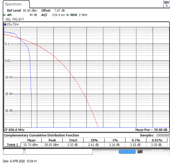
EGPRS850-190-8-PASS
