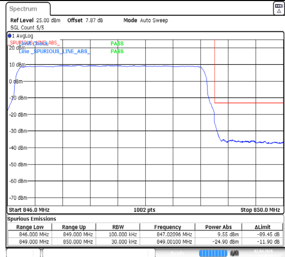
Band26(824-849)-3MHz-QPSK-27025-1RB#0-PASS
