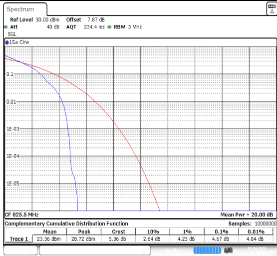
Band26(824-849)-3MHz-QPSK-26805-1RB#0-PASS
