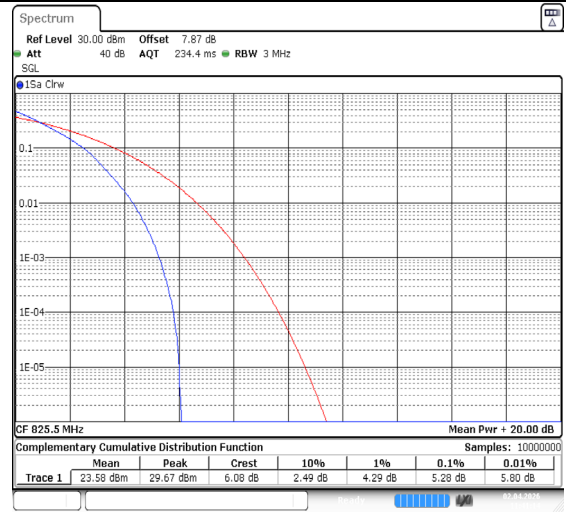
Band26(824-849)-3MHz-QPSK-26805-15RB#0-PASS
