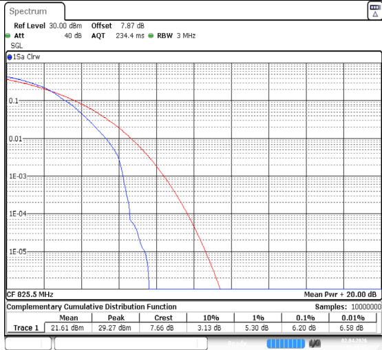
Band26(824-849)-3MHz-QPSK-26805-1RB#0-PASS
