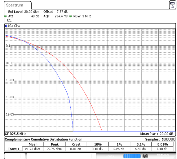
Band26(824-849)-3MHz-QPSK-26805-15RB#0-PASS
