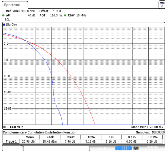
Band26(824-849)-10MHz-QPSK-26990-1RB#0-PASS
