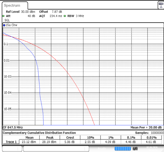
Band26(824-849)-3MHz-QPSK-27025-1RB#0-PASS
