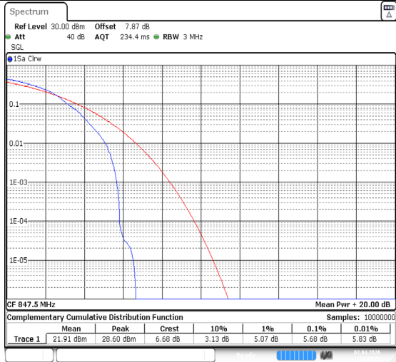
Band26(824-849)-3MHz-QPSK-27025-1RB#0-PASS
