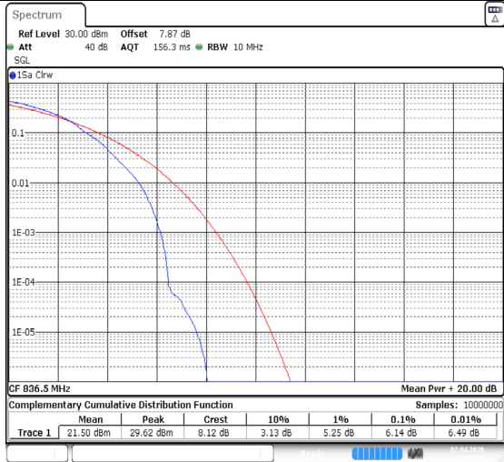
Band26(824-849)-10MHz-QPSK-26915-1RB#0-PASS
