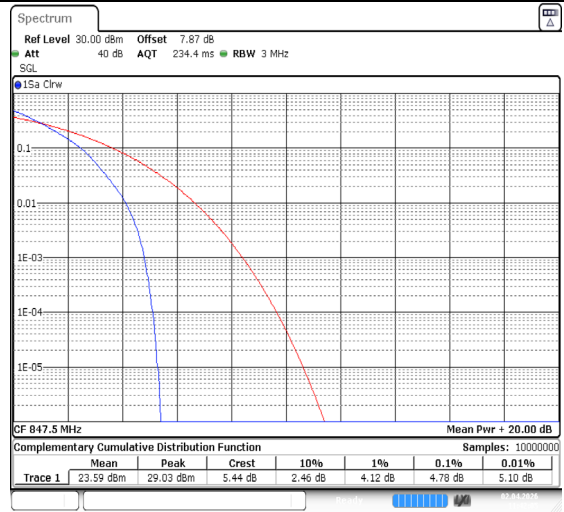
Band26(824-849)-3MHz-QPSK-27025-15RB#0-PASS
