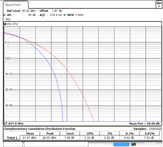
Band26(824-849)-3MHz-QPSK-27025-15RB#0-PASS
