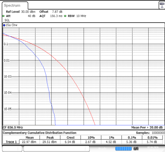
Band26(824-849)-10MHz-QPSK-26915-1RB#0-PASS
