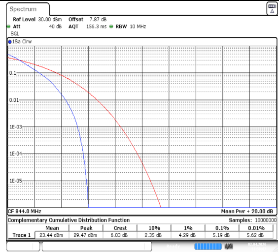
Band26(824-849)-10MHz-QPSK-26990-50RB#0-PASS
