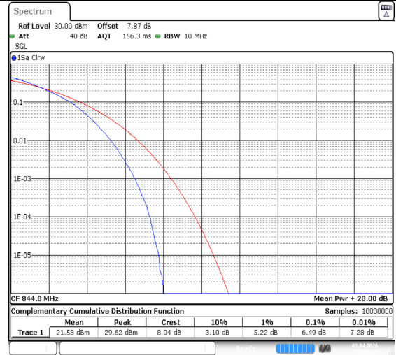
Band26(824-849)-10MHz-QPSK-26990-50RB#0-PASS
