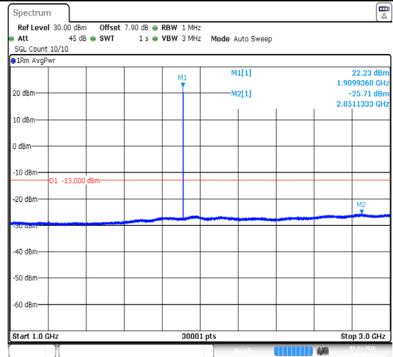
GSM1900-810-0-1000~3000MHz-PASS
