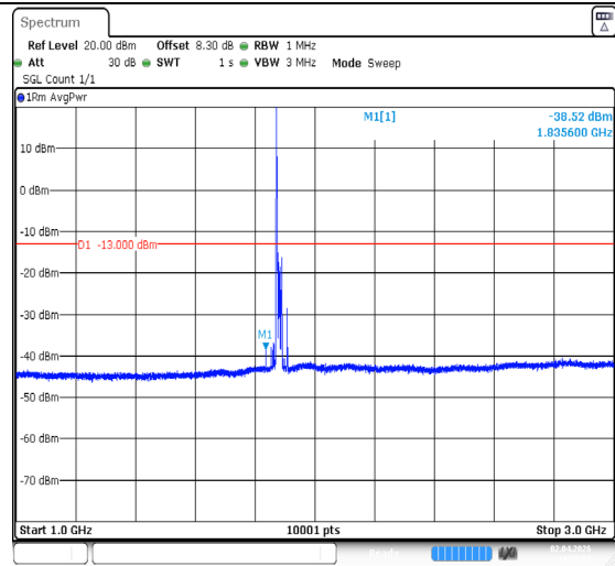
Band2-20MHz-QPSK-18900-1RB#0-1000~3000-PASS
