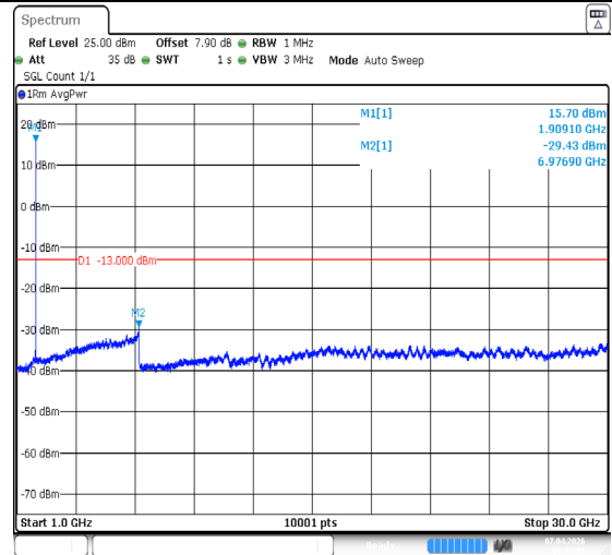
Band2-9538-1000~30000MHz-PASS
