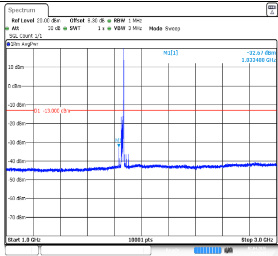
Band2-20MHz-QPSK-18700-1RB#99-1000~3000-PASS
