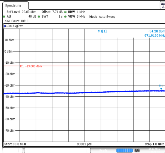
EGPRS1900-810-2-30~1000MHz-PASS
