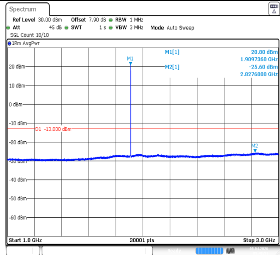
EGPRS1900-810-2-1000~3000MHz-PASS
