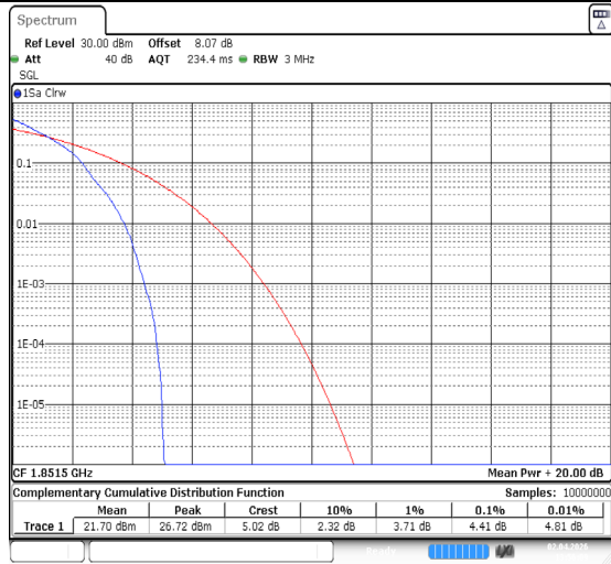
Band2-3MHz-QPSK-18615-1RB#0-PASS
