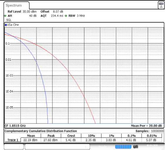
Band2-3MHz-QPSK-18615-15RB#0-PASS
