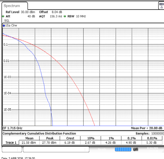
Band4-10MHz-QPSK-20000-1RB#0-PASS
