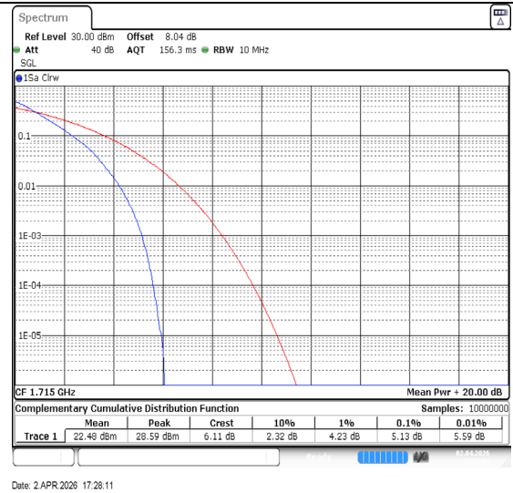
Band4-10MHz-QPSK-20000-50RB#0-PASS
