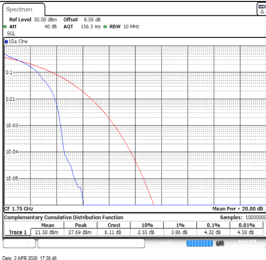
Band4-10MHz-QPSK-20350-1RB#0-PASS
