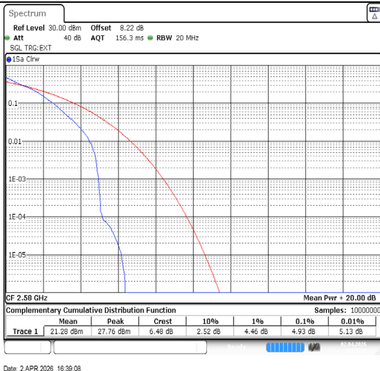
Band38-20MHz-QPSK-37850-1RB#0-PASS
