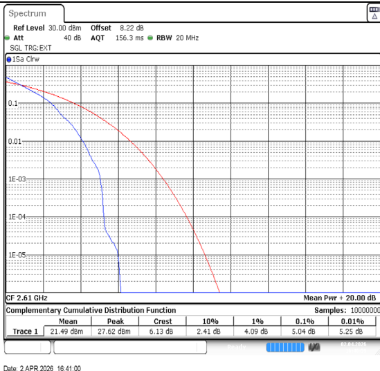
Band38-20MHz-QPSK-38150-1RB#0-PASS
