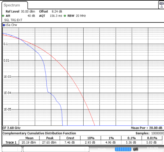
Band41-20MHz-QPSK-41490-1RB#0-PASS
