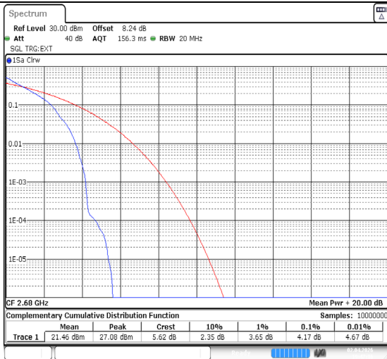
Band41-20MHz-QPSK-41490-1RB#0-PASS
