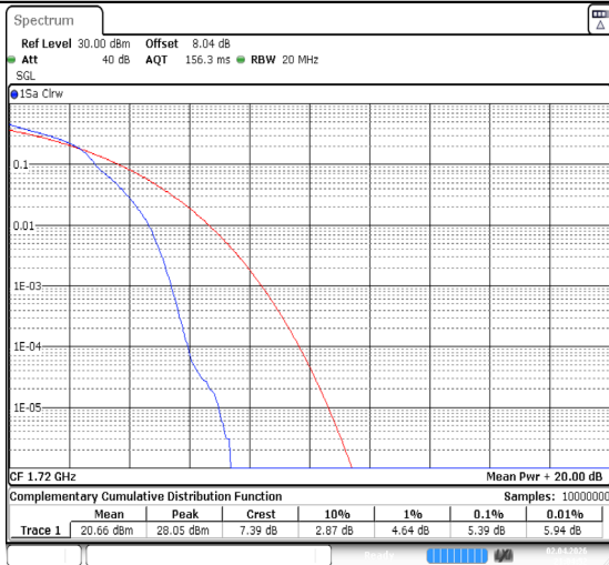
Band66-20MHz-QPSK-132072-1RB#0-PASS
