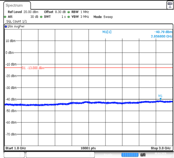
Band26(824-849)-1.4MHz-QPSK-26797-1RB#0-1000~3000-PASS
