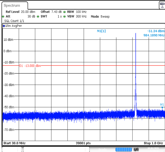
Band26(824-849)-1.4MHz-QPSK-26797-6RB#0-30~1000-PAS S
