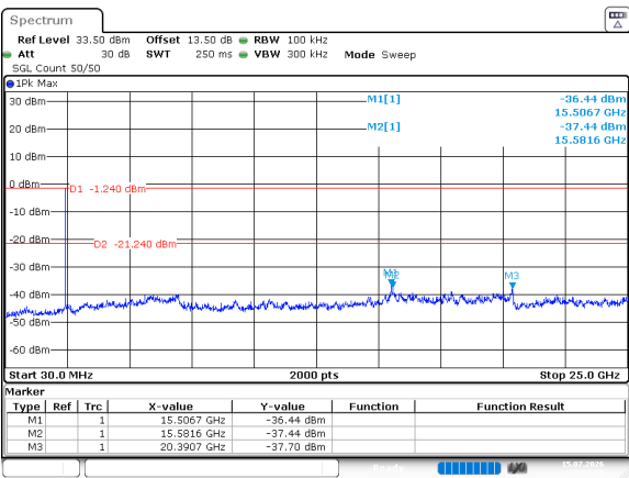
802.11b_2437MHz
