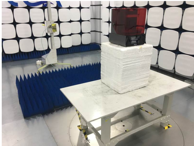
Above 1GHz:
