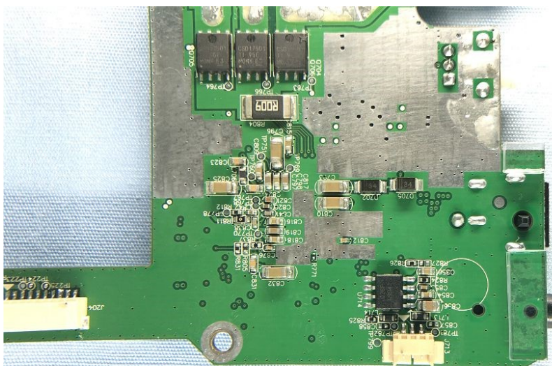
(6) EUT Photo
