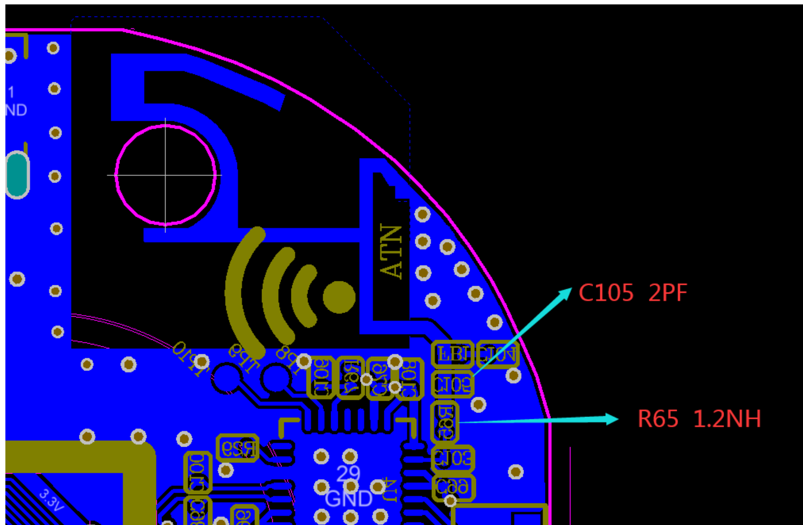
新天线产品匹配电路图
