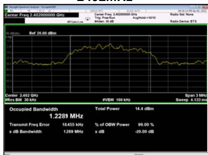
2402MHz
