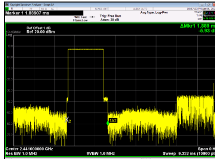
DH3
