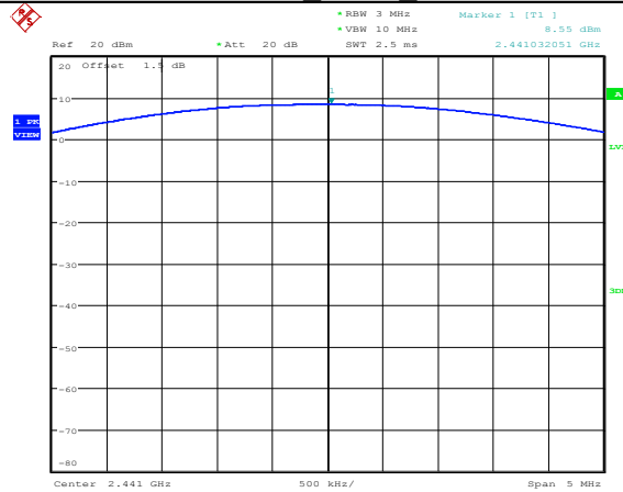
DH5 ANT1 2441
