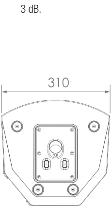
Vista inferior
