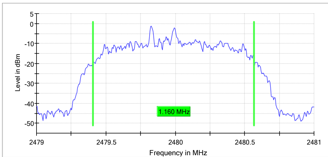
3DH5 Ant1 2480
