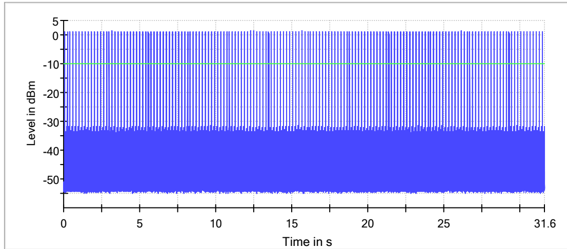
3DH5_Ant1_Hop
