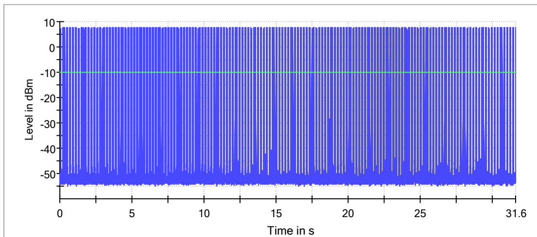
DH1_Ant1_Hop
