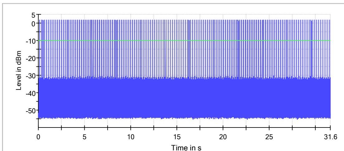
DH3_Ant1_Hop
