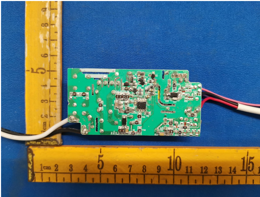
Fig.6 (Model:18SCO-KA)
