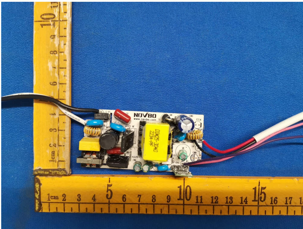
Fig.7 (Model:18SCO-KA)
