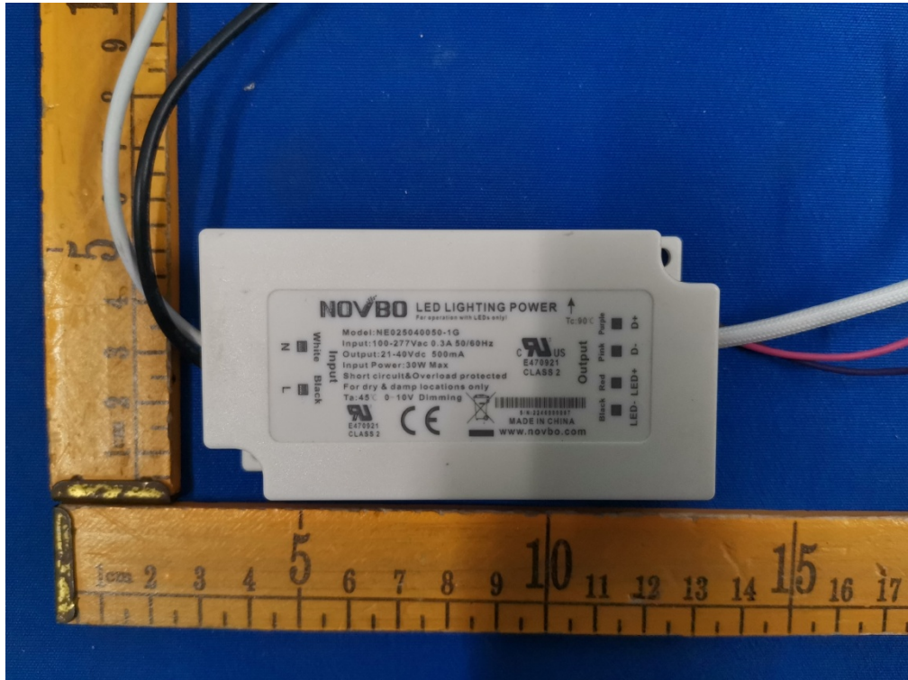
Fig.4 (Model:18SCO-KA)
