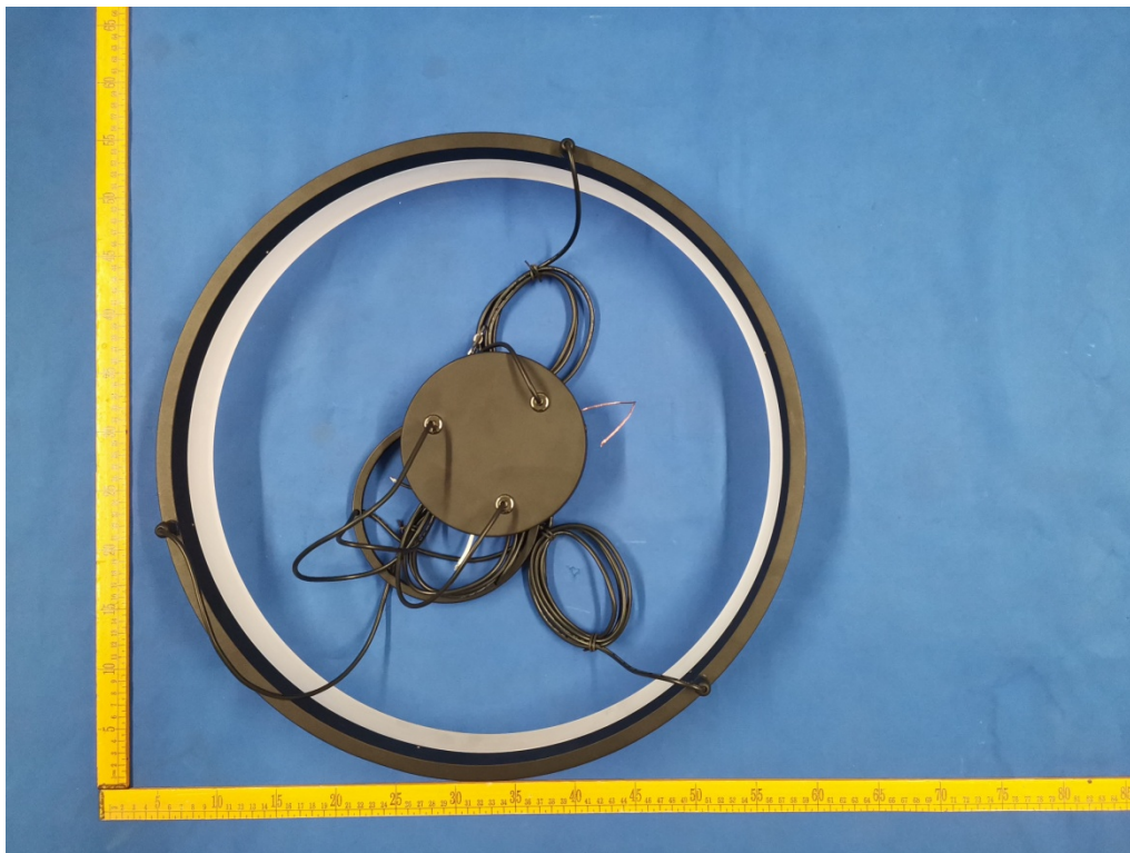
Fig.1(Model: OPDT-OPC)
