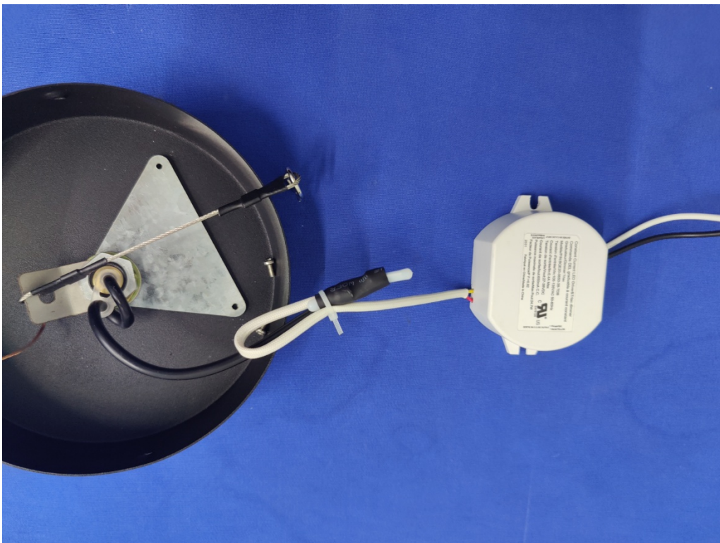
Fig.4(Model: OPTD1-AR)
