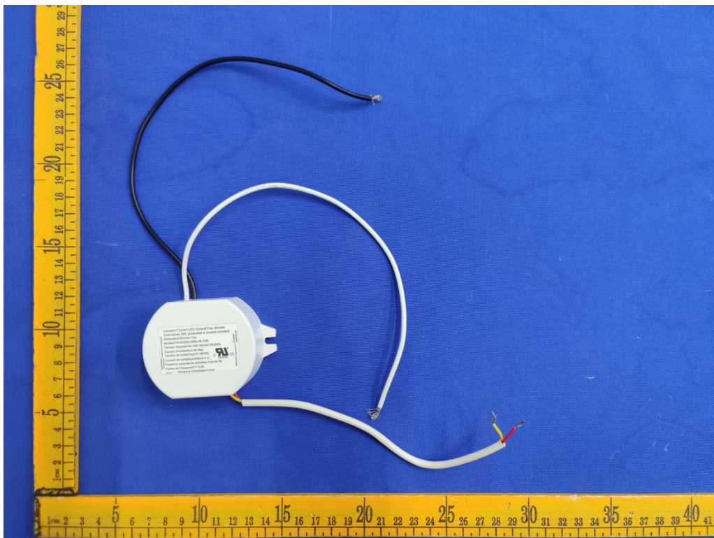
Fig.6(Model: OPTD1-AR)
