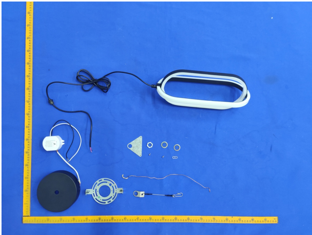
Fig.5(Model: OPTD1-AR)
