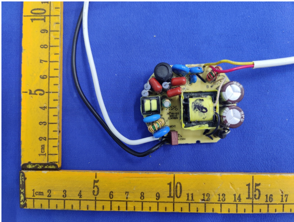
Fig.9(Model: OPTD1-AR)
