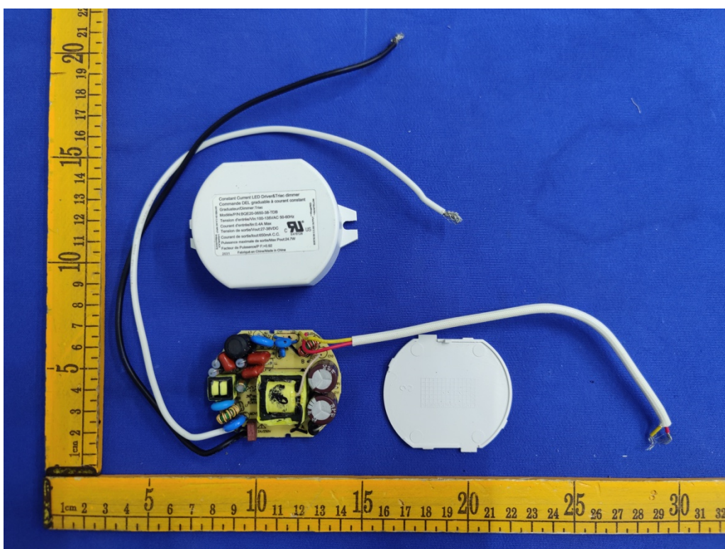
Fig.8(Model: OPTD1-AR)
