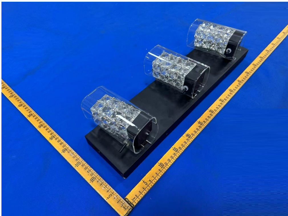
Fig.4(Model: VAN3-CC5C )
