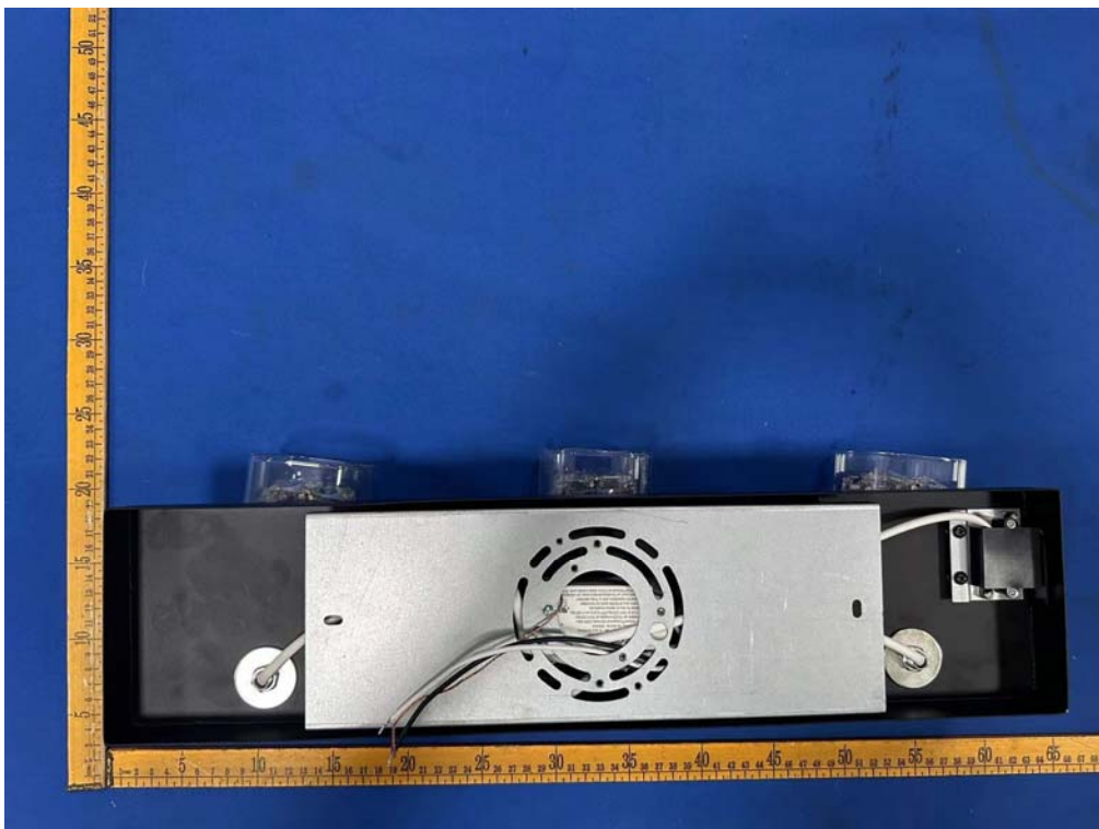
Fig.2(Model: VAN3-CC5C )
