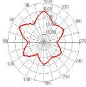
2400.000MHz E2
