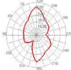
2410.000MHz H
