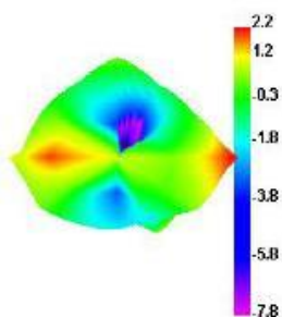
2410.000MHz
