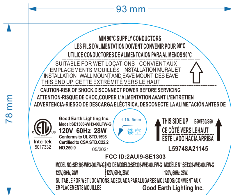
铭牌贴纸 白色机,白底黑字
