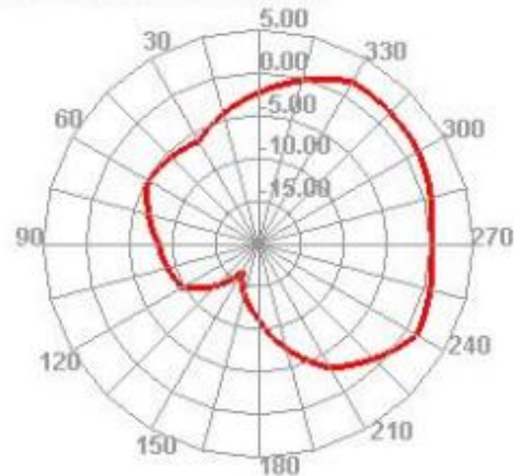
2500.000MHz E2
