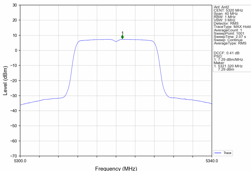
802.11a_HCH_5320MHz_Ant2_NTNV
