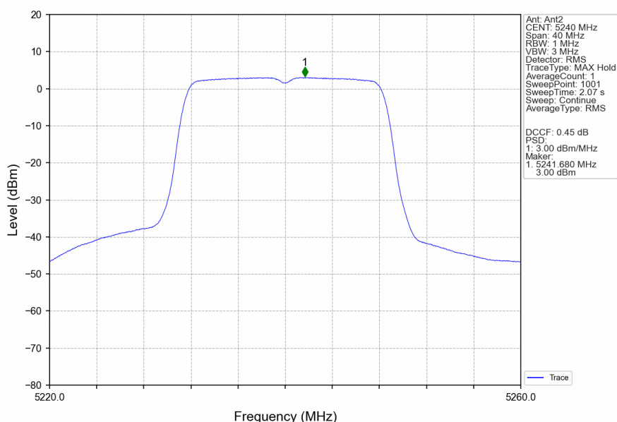
802.11a_HCH_5240MHz_Ant2_NTNV
