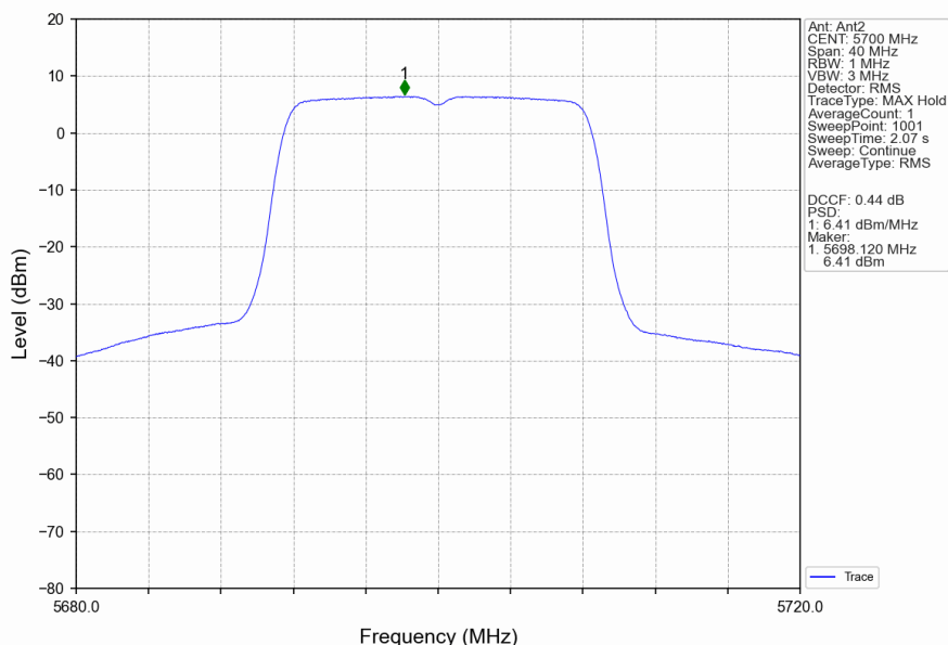
802.11a_HCH_5700MHz_Ant2_NTNV
