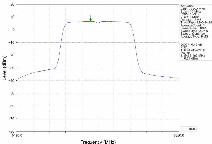
802.11a_LCH_5500MHz_Ant2_NTNV
