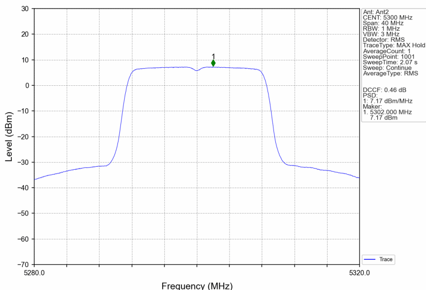
802.11a_MCH_5300MHz_Ant2_NTNV
