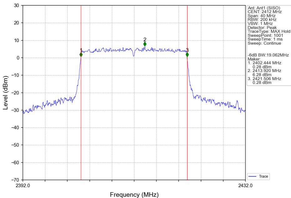
802.11ax(HEW20)_LCH_2412MHz_SU_/_Ant1 (SISO)_NTNV
