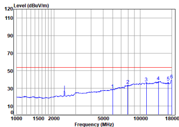
11ax_20M_TX_CH_06_Vertical-Avg
