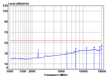
11ax_20M_TX_CH_06_Horizontal-Avg
