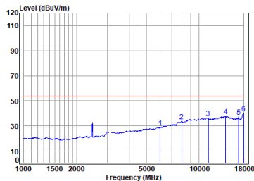
11ax_20M_TX_CH_11_Vertical-Avg
