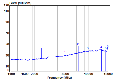
BLE_1M_TX_CH_39_Horizontal-Avg
