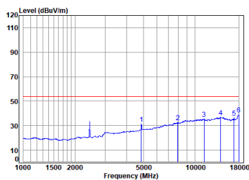
11n_20M_TX_CH_06_Horizontal-Avg
