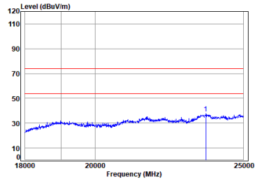
11b_TX_CH_01_Vertical
