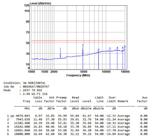
11b_TX_CH_06_Horizontal-Avg
