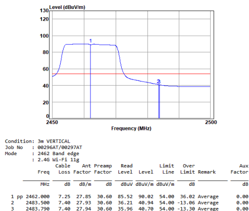
11g_TX_CH_11_Vertical-Avg
