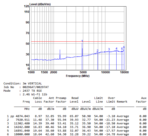
11b_TX_CH_06_Vertical-Avg
