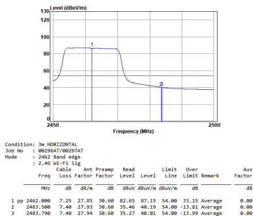
11g_TX_CH_11_Horizontal-Avg
