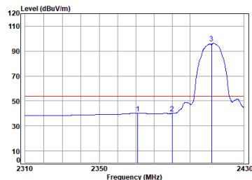
11b_TX_CH_01_Vertical-Avg
