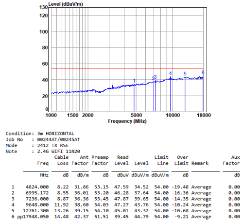
11n_20M_TX_CH_01_Horizontal-Avg
