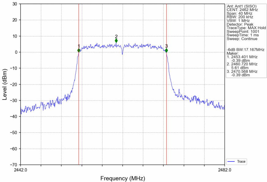
802.11n(HT20)_HCH_2462MHz_Ant1 (SISO)_NTNV
