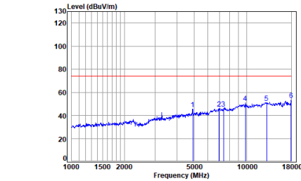
11n_20M_TX_CH_11_Vertical-Peak
