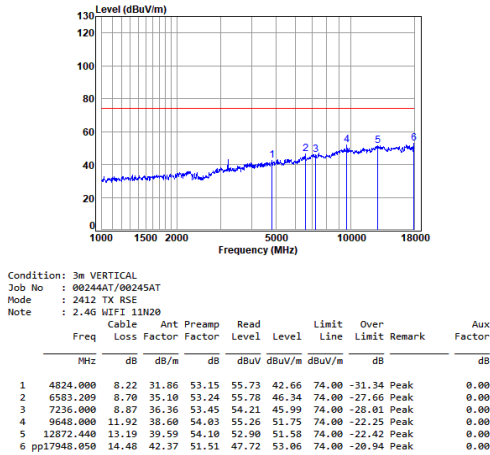
11n_20M_TX_CH_01_Vertical-Peak
