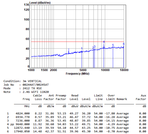
11n_20M_TX_CH_01_Vertical-Avg
