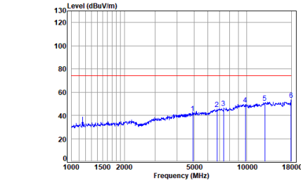
11n_20M_TX_CH_11_Horizontal-Peak
