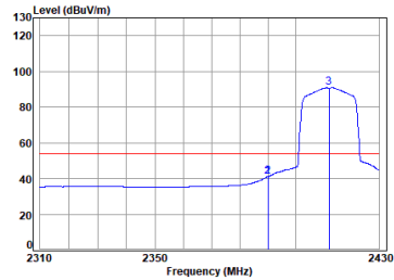
11ax_20M_TX_CH_01_Vertical-Avg
