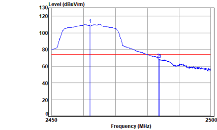
11n_HT(20M)_TX_CH_11_Horizontal-Peak
