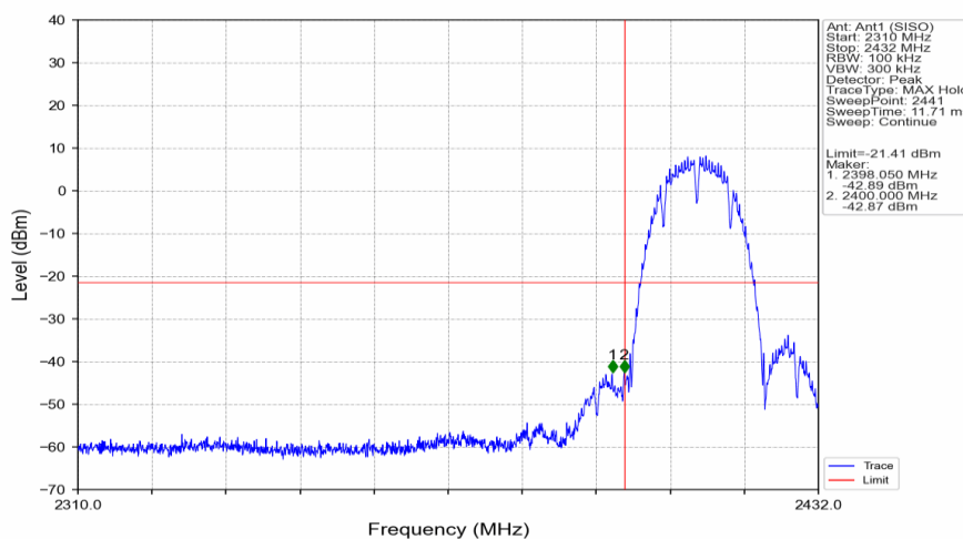
802.11b_LCH_2412MHz_Ant1 (SISO)_NTNV
