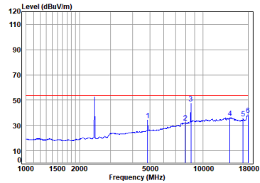
11b_TX_CH_06_Vertical-Avg
