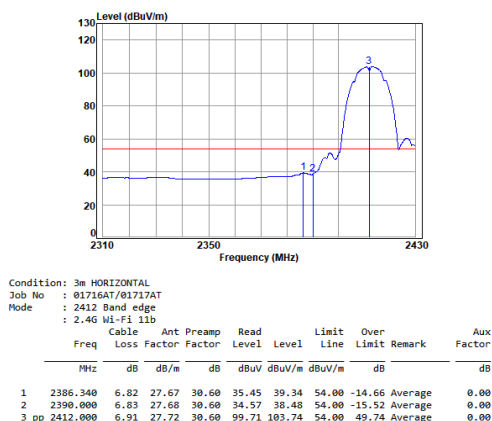
11b_TX_CH_01_Horizontal-Avg
