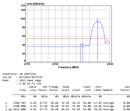
11b_TX_CH_01_Vertical-Avg
