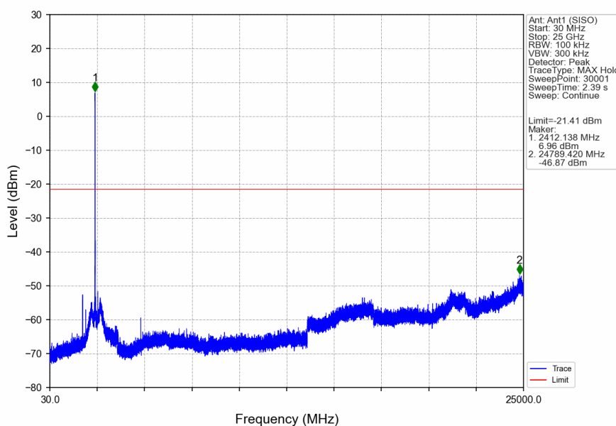
802.11b_LCH_2412MHz_Ant1 (SISO)_NTNV
