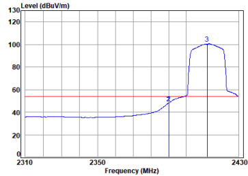
11ax_20M_TX_CH_01_Horizontal-Avg
