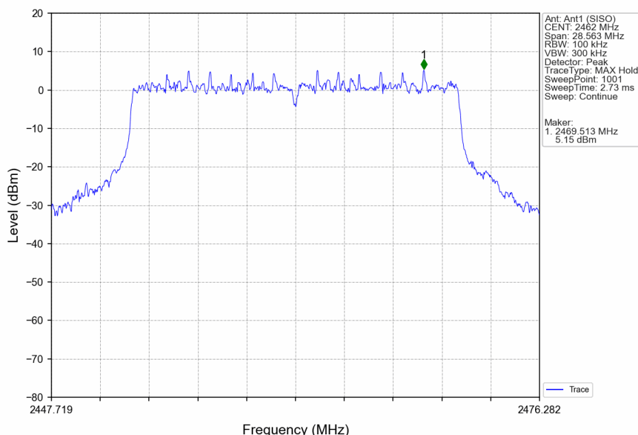
802.11ax(HEW20)_HCH_2462MHz_RU242_Left_Ant1 (SISO)_NTNV
