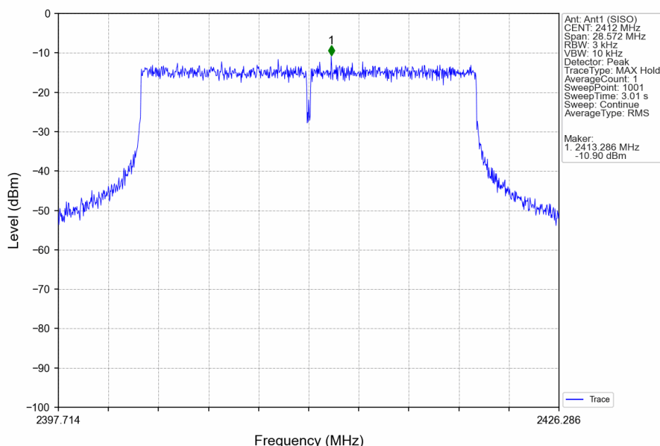
802.11ax(HEW20)_LCH_2412MHz_RU242_Left_Ant1 (SISO)_NTNV
