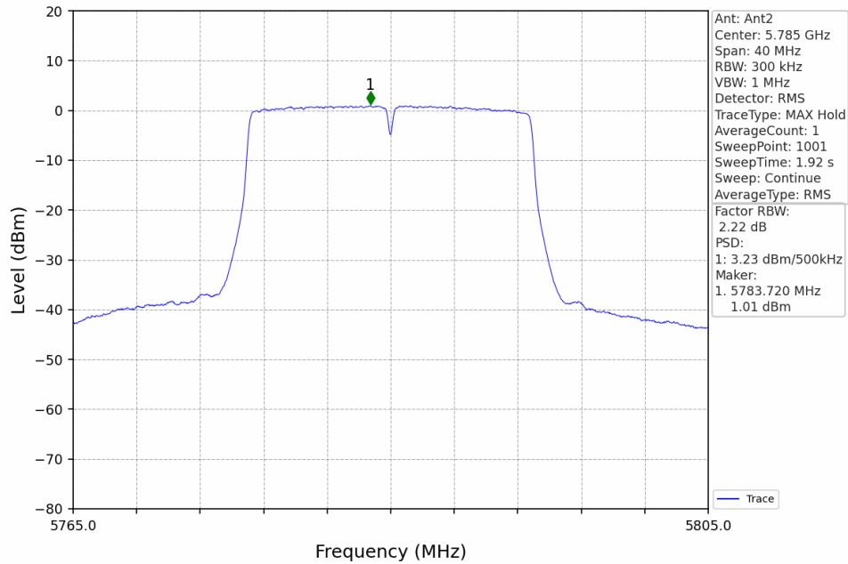
802.11n(HT20)_MCH_5785MHz_MIMO_NTNV
