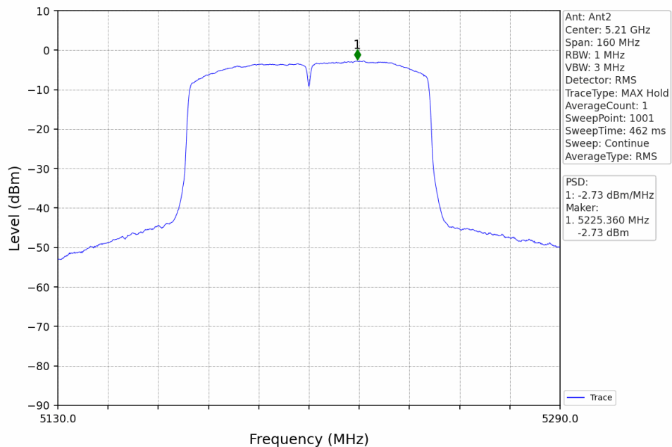
802.11ac(VHT80)_MCH_5210MHz_Ant2_NTNV
