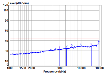
BLE_2M_TX_CH_39_Vertical-Avg
