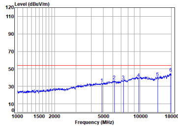
BLE_2M_TX_CH_19_Horizontal-Avg
