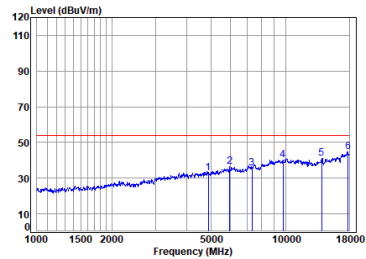
BLE_2M_TX_CH_19_Horizontal-Avg
