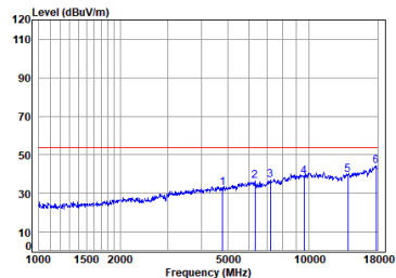
BLE_2M_TX_CH_00_Vertical-Avg
