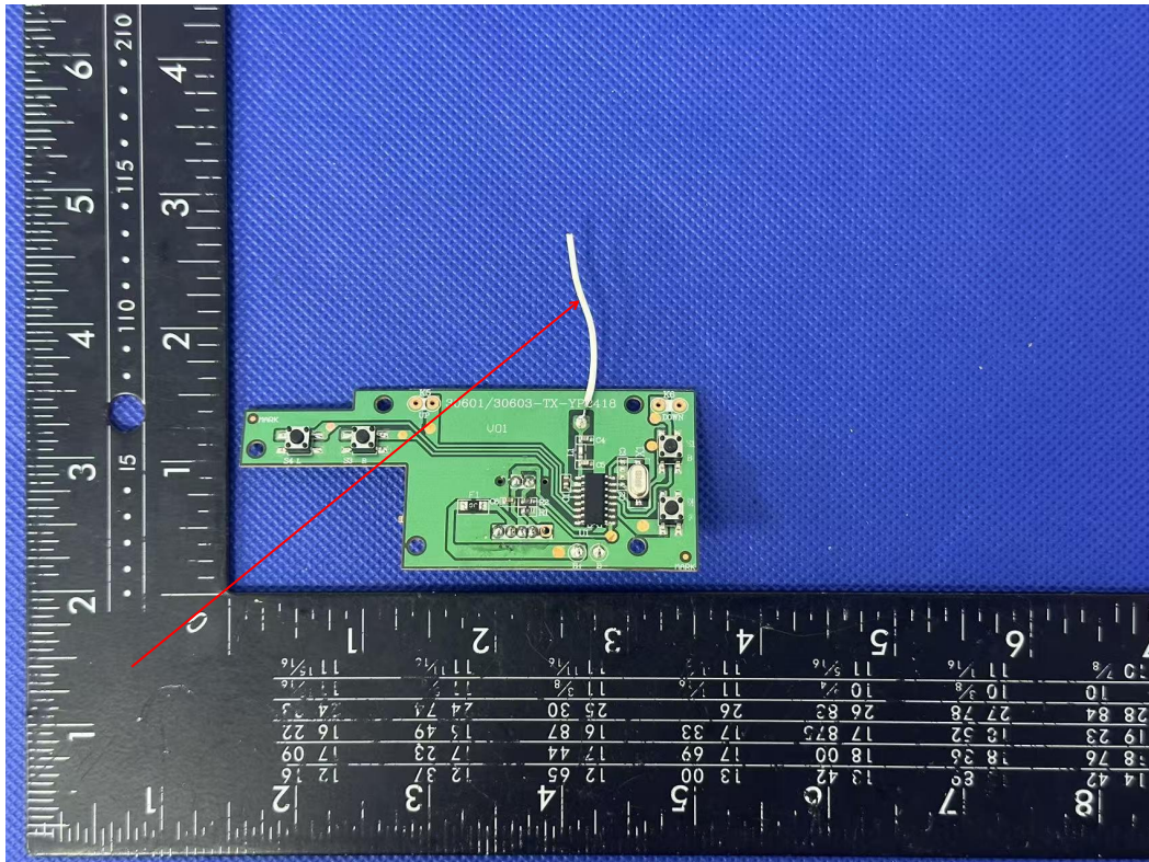
2.4G ANT
