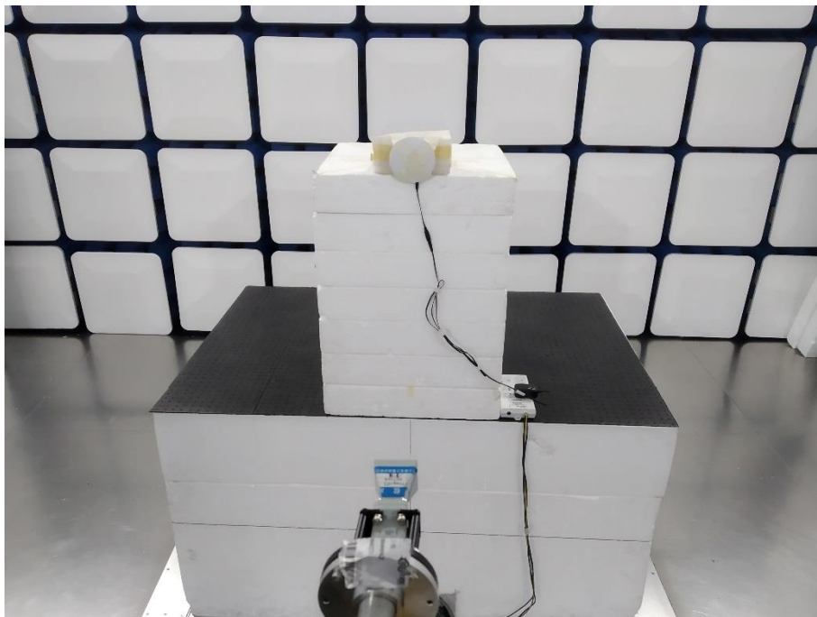
Above 18GHz
