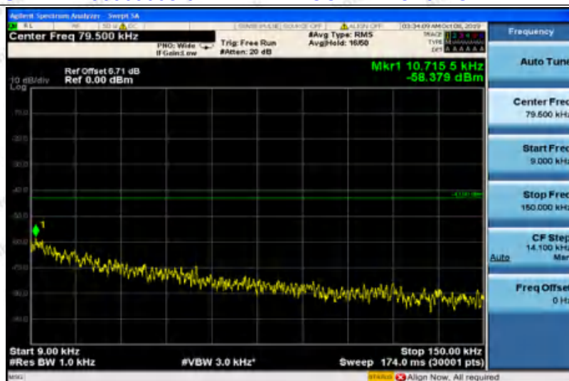
GPRS1900-810-0.009~0.15
