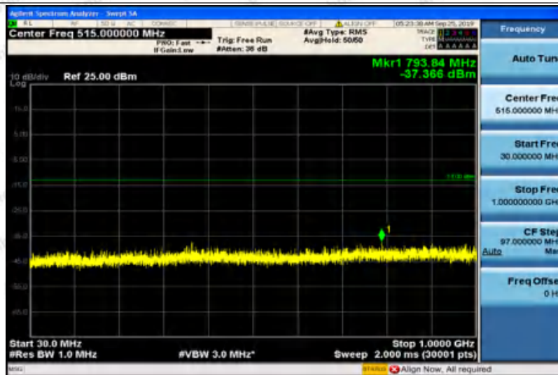
Band2-15MHz-16QAM-18675-1RB#0-Range2:1000~5000MHz
