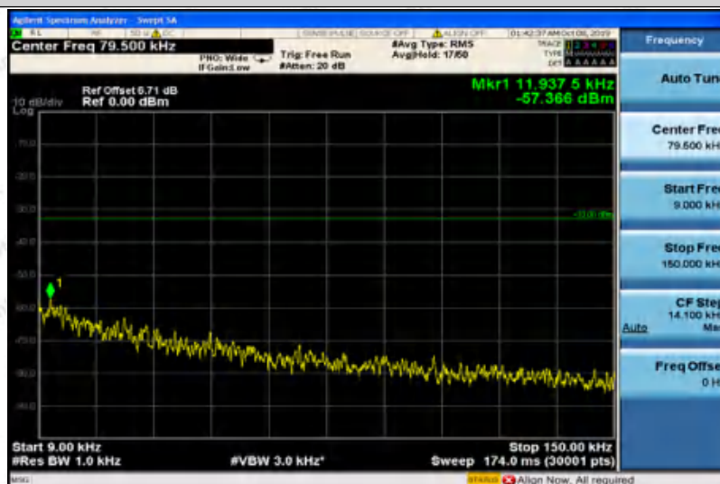
GPRS850-190-0.009~0.15
