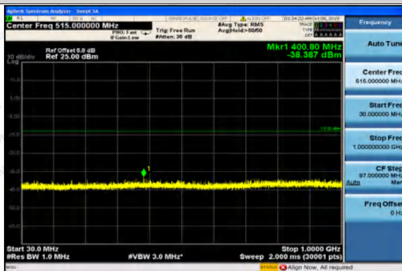
GPRS1900-810-30~1000
