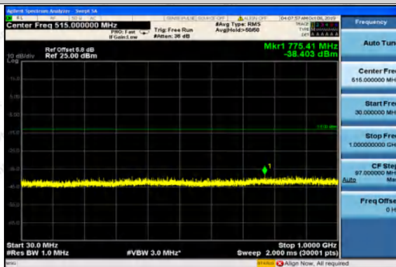
EGPRS1900-810-30~1000
