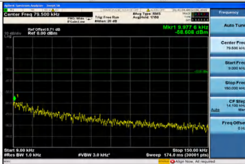
GPRS850-128-0.009~0.15
