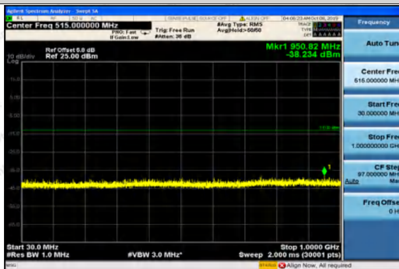
EGPRS1900-661-30~1000
