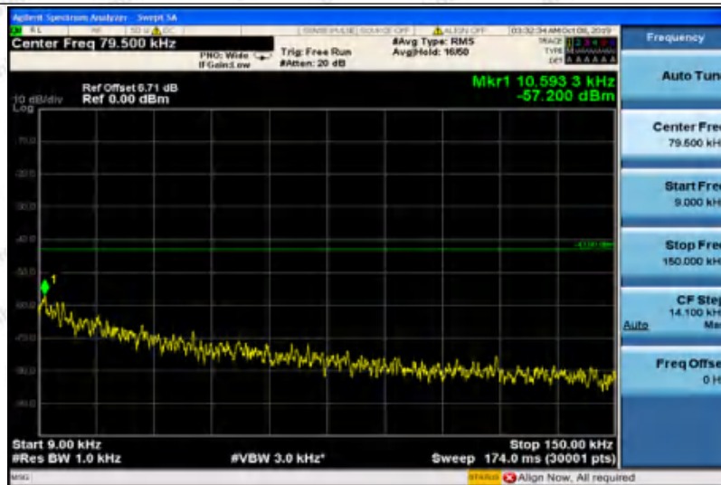
GPRS1900-661-0.009~0.15
