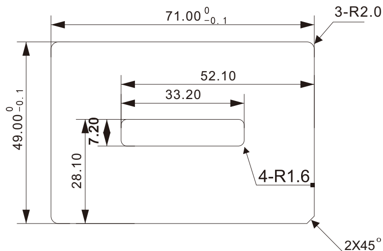
(尺寸图)
