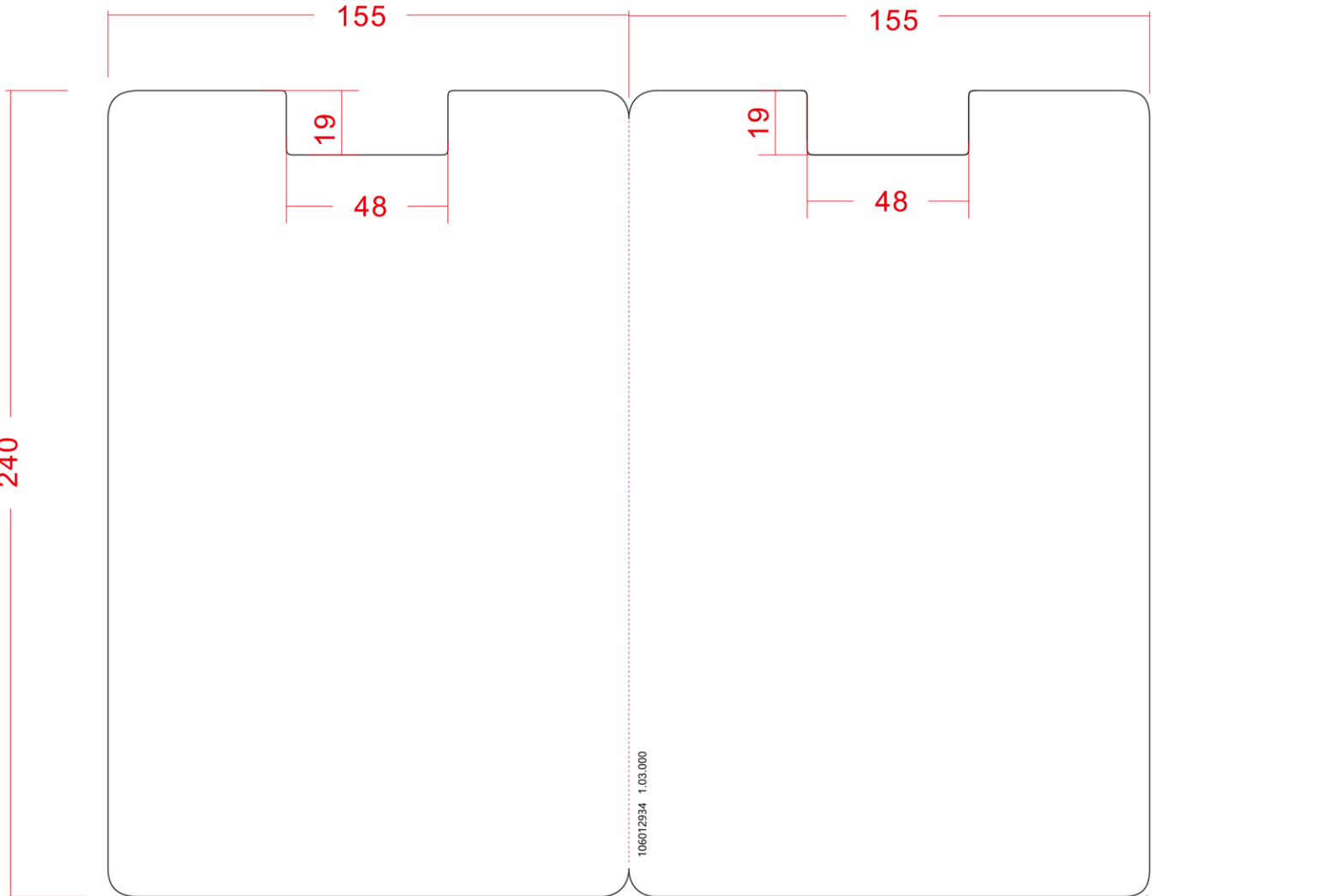
刀模图
