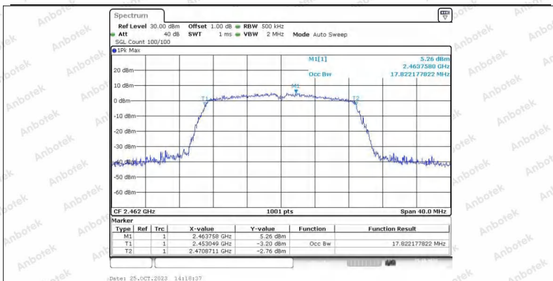
11N20SISO_Ant2_2462
