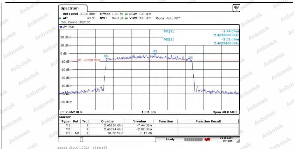
11AX20SISO_Ant2_2462
