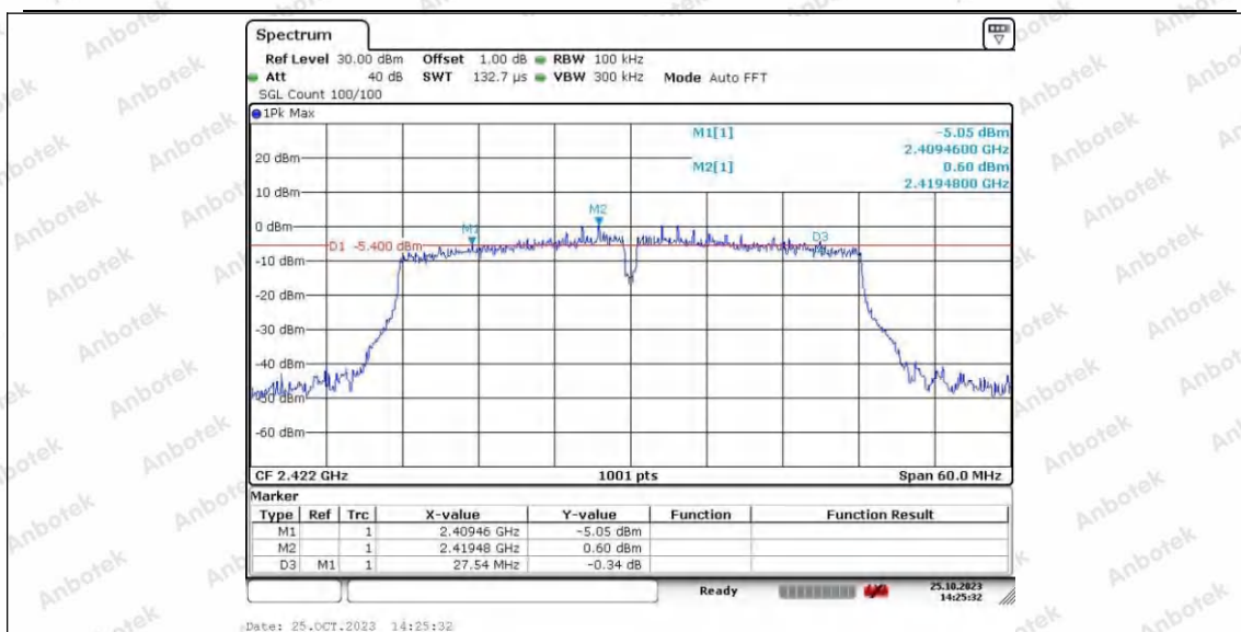
11N40SISO_Ant2_2422
