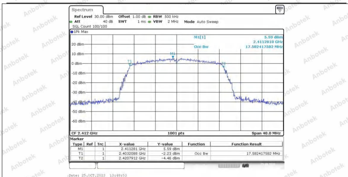
11N20SISO_Ant2_2412
