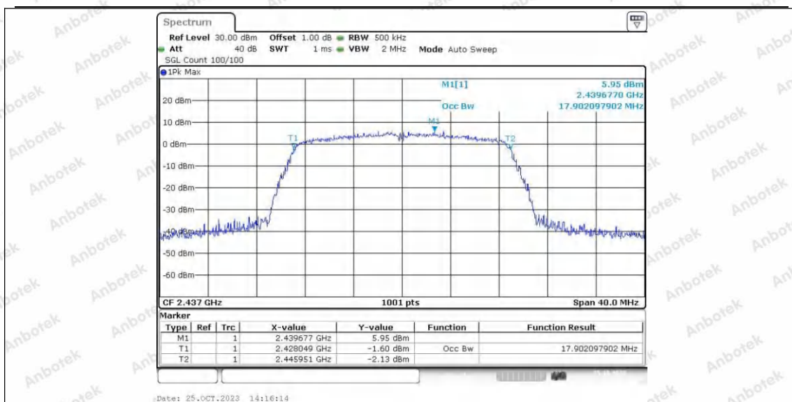
11N20SISO_Ant2_2437
