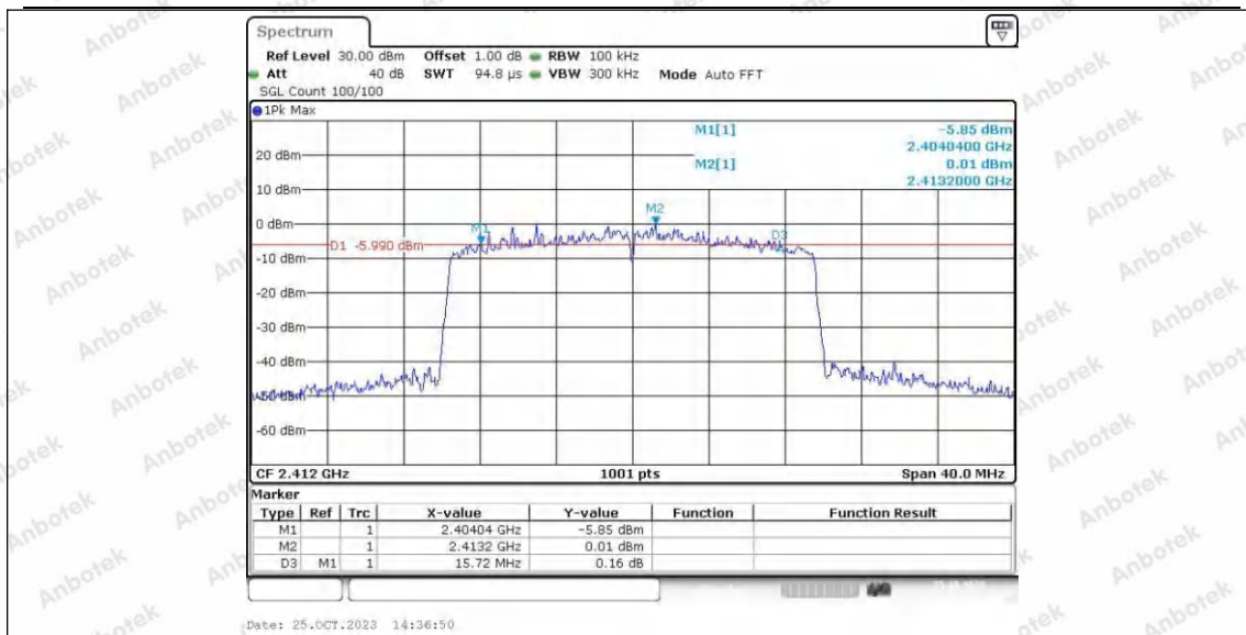
11AX20SISO_Ant2_2412
