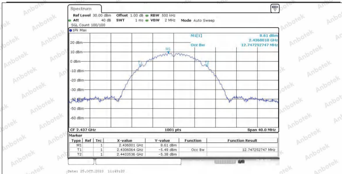
11B_Ant2_2437
