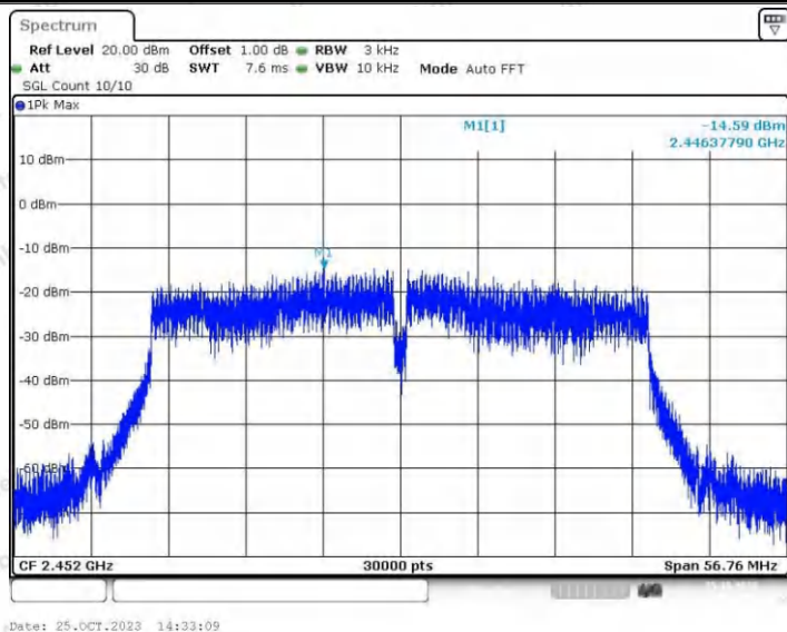
11N40SISO_Ant2_2452
