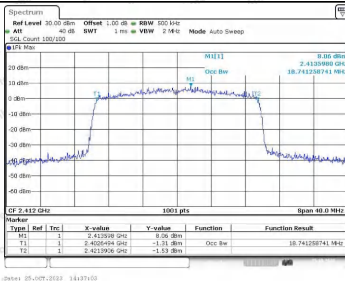
11AX20SISO_Ant2_2412
