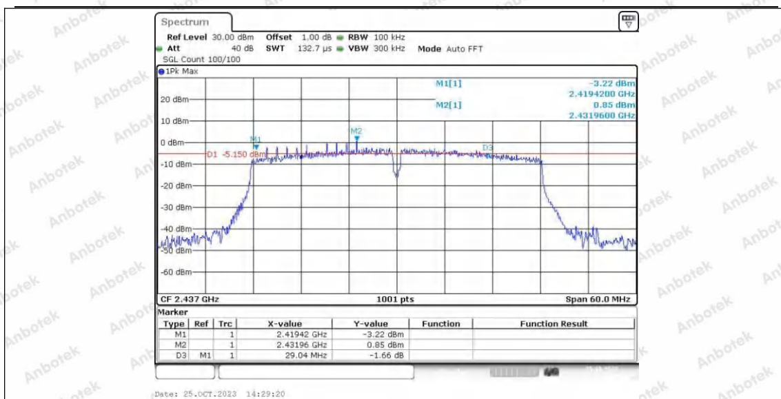
11N40SISO_Ant2_2437
