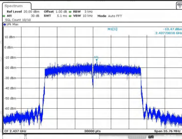
11AX20SISO_Ant2_2437
