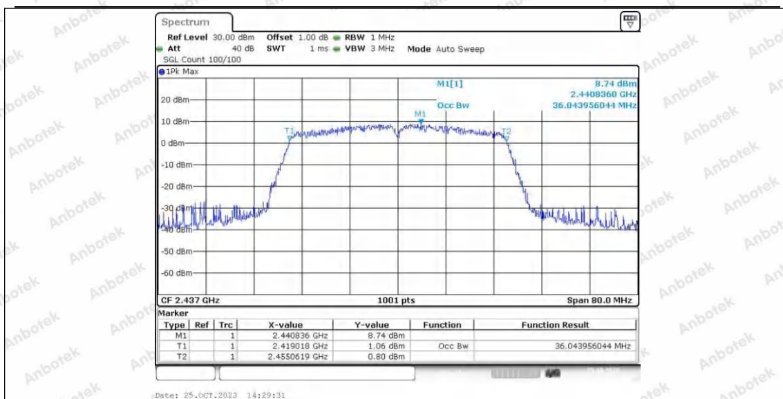
11N40SISO_Ant2_2437
