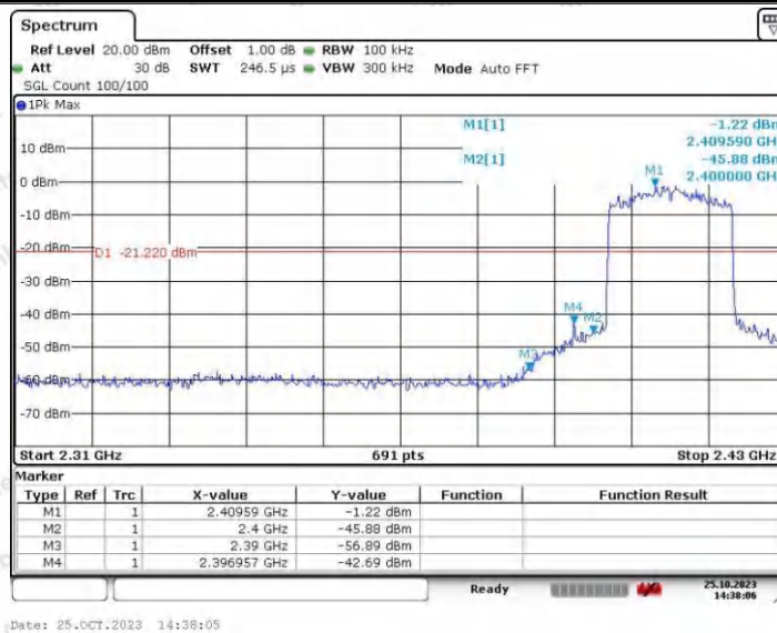
11AX20SISO_Ant2_Low_2412
