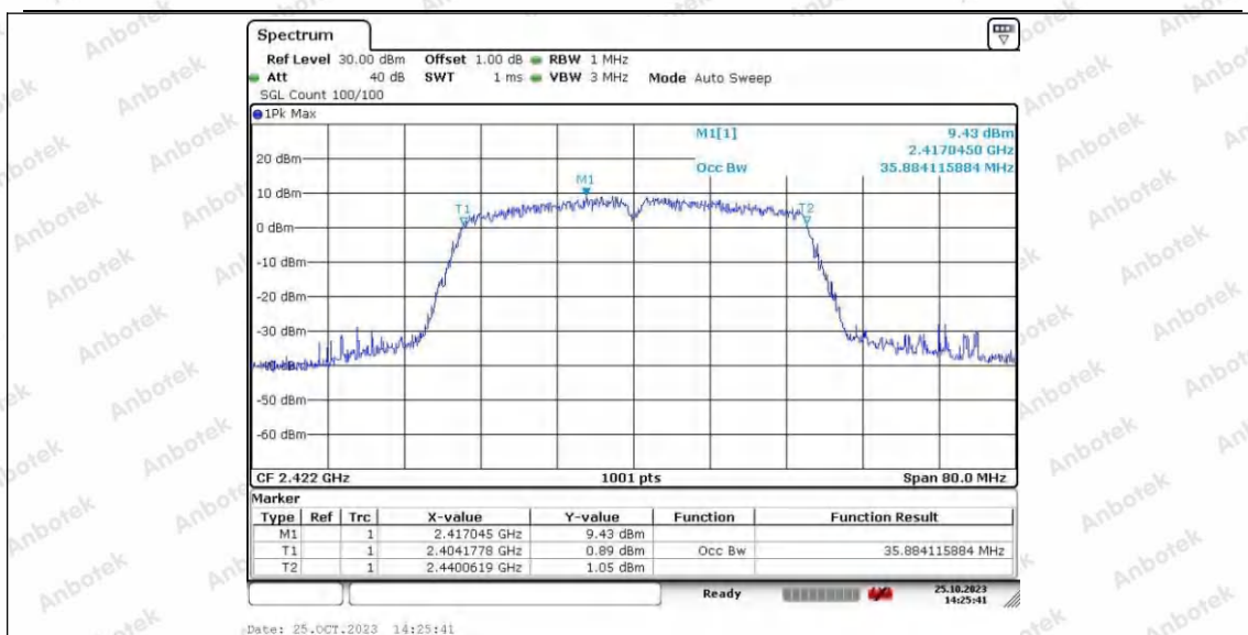
11N40SISO_Ant2_2422
