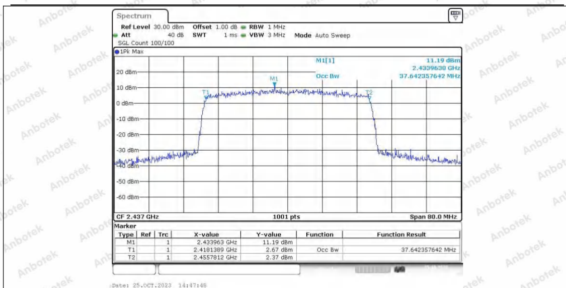
11AX40SISO_Ant2_2437
