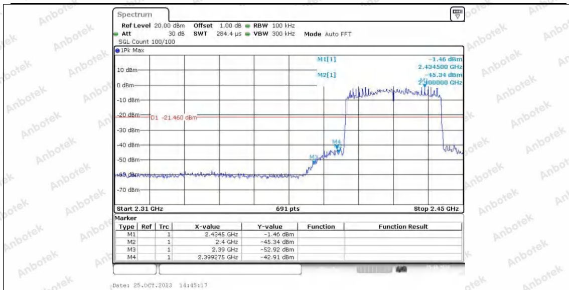
11AX40SISO_Ant2_Low_2422
