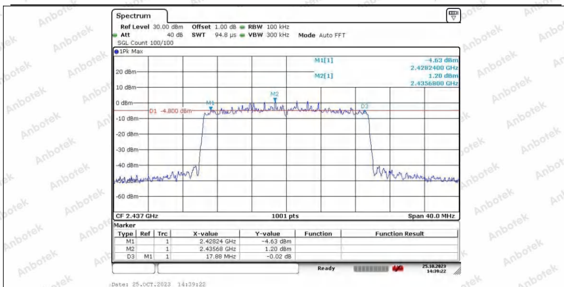
11AX20SISO_Ant2_2437
