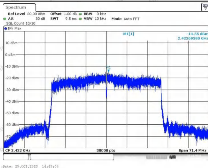
11AX40SISO_Ant2_2422
