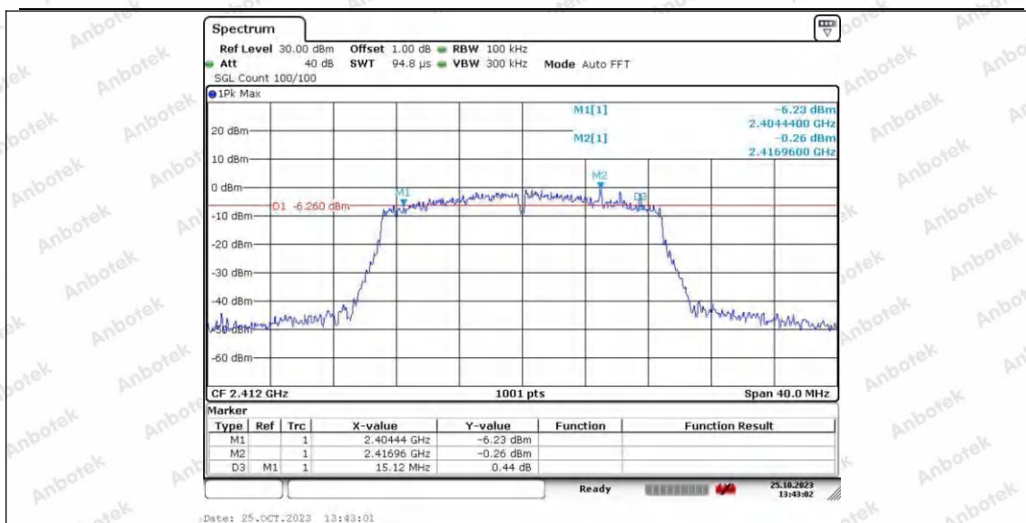
11N20SISO_Ant2_2412
