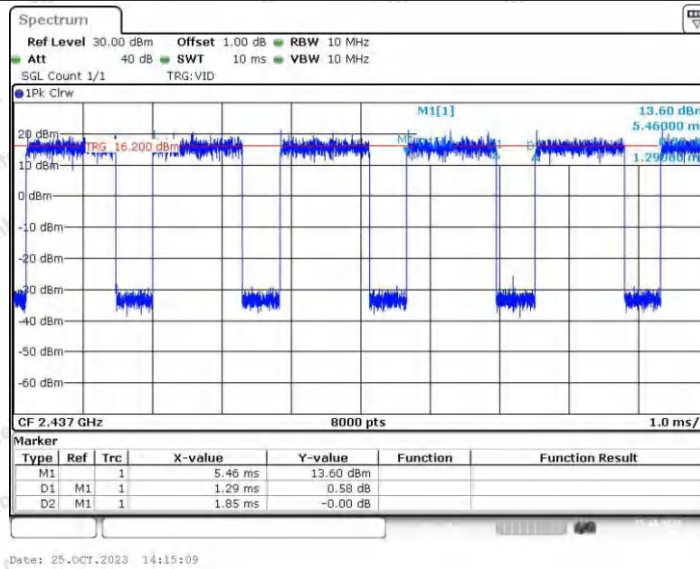
11N20SISO_Ant2_2437
