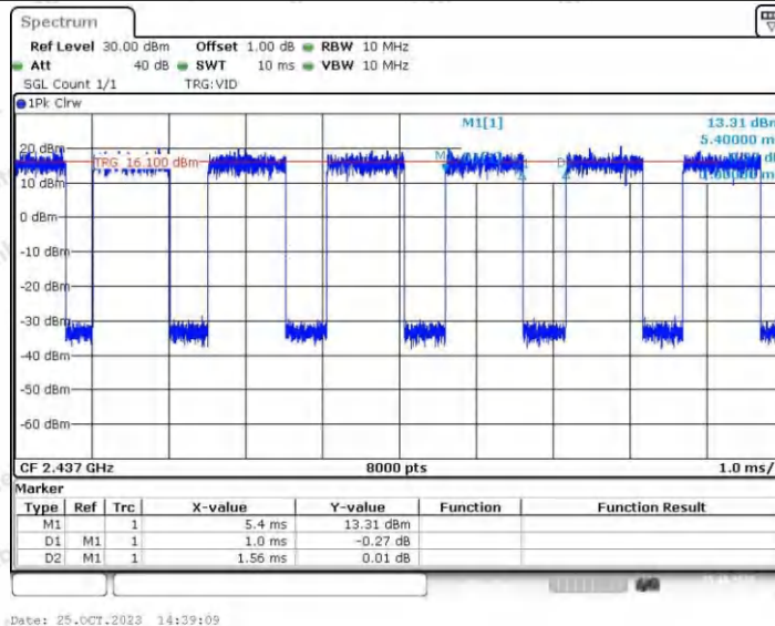
11AX20SISO_Ant2_2437
