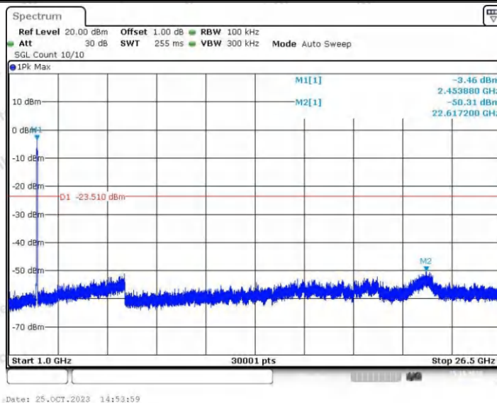
11AX40SISO_Ant2_2452_0~Reference
