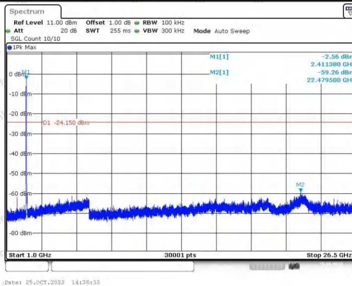
11AX20SISO_Ant2_2412_0~Reference
