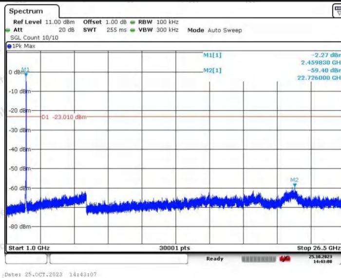
11AX20SISO_Ant2_2462_0~Reference
