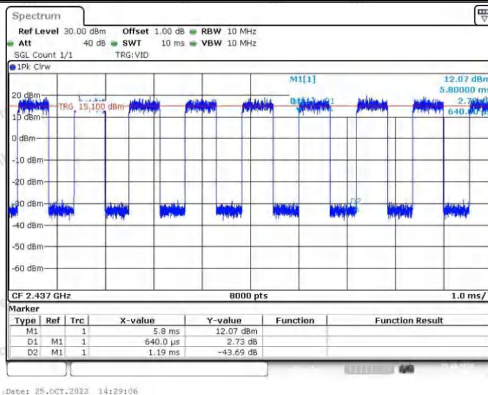
11N40SISO_Ant2_2437
