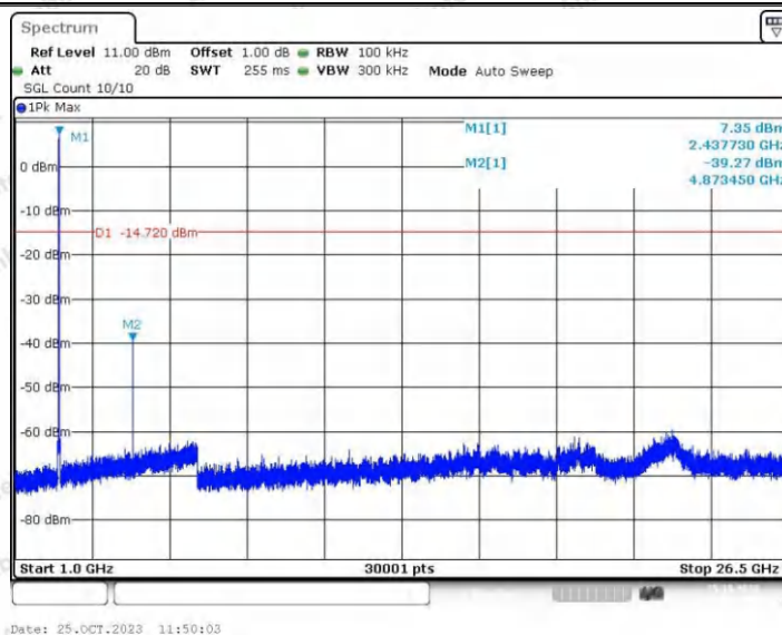
11B_Ant2_2437_0~Reference
