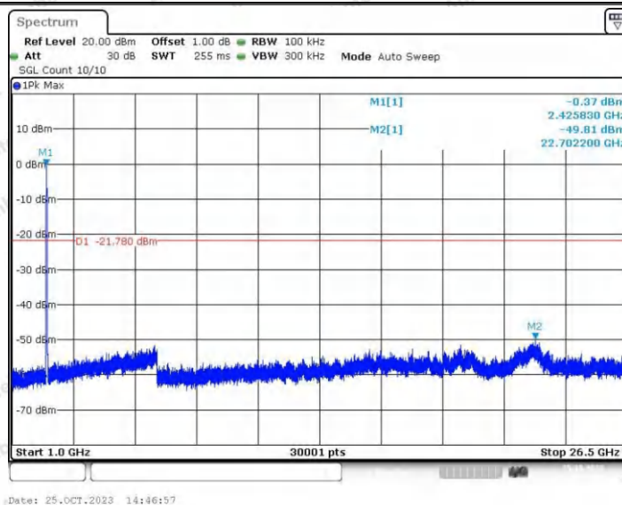
11AX40SISO_Ant2_2422_0~Reference
