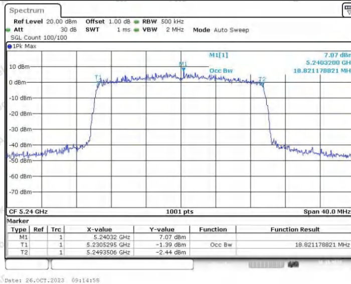
11AX20SISO_Ant2_5240
